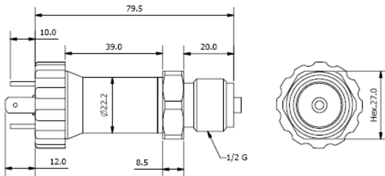
DIN EN 175301-803 with 27mm Hex.
